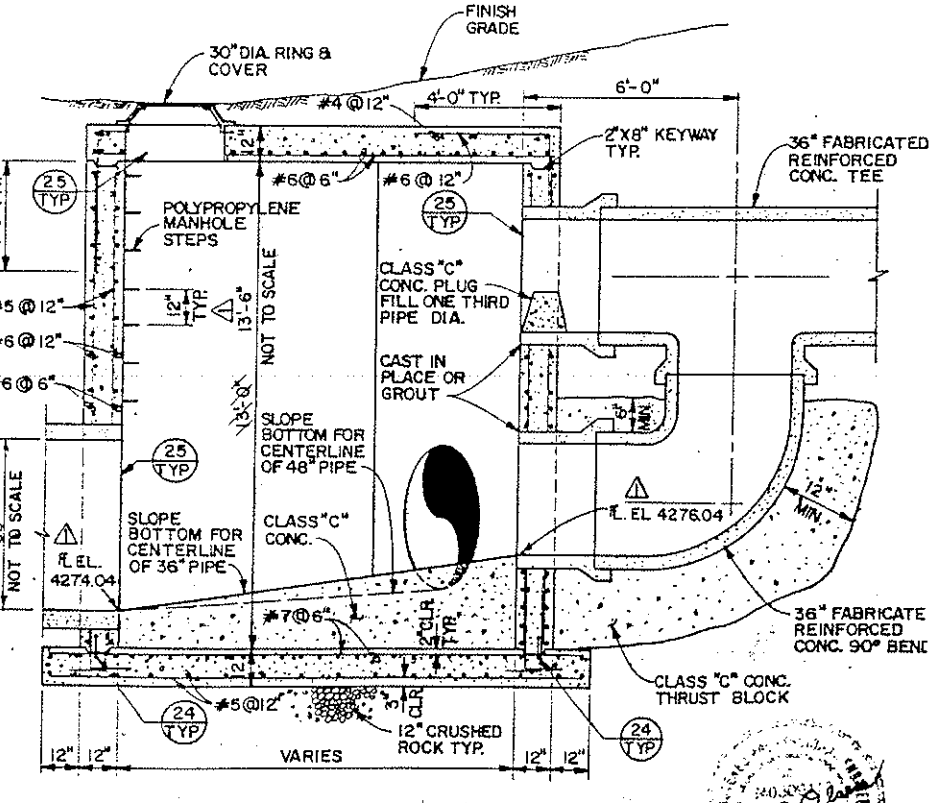
F SECTION SCALE: 3/8" = 1'-0"
