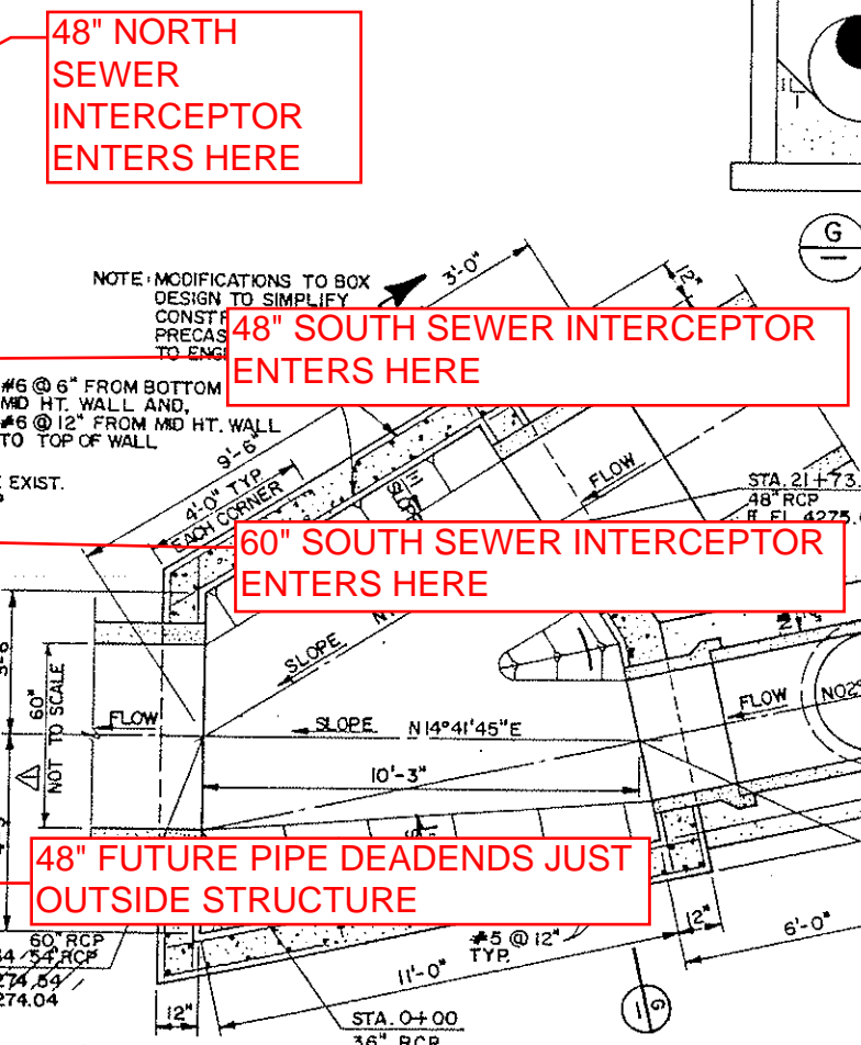
E JUNCTION BOX SCALE: 3/8" = 1'-0"
