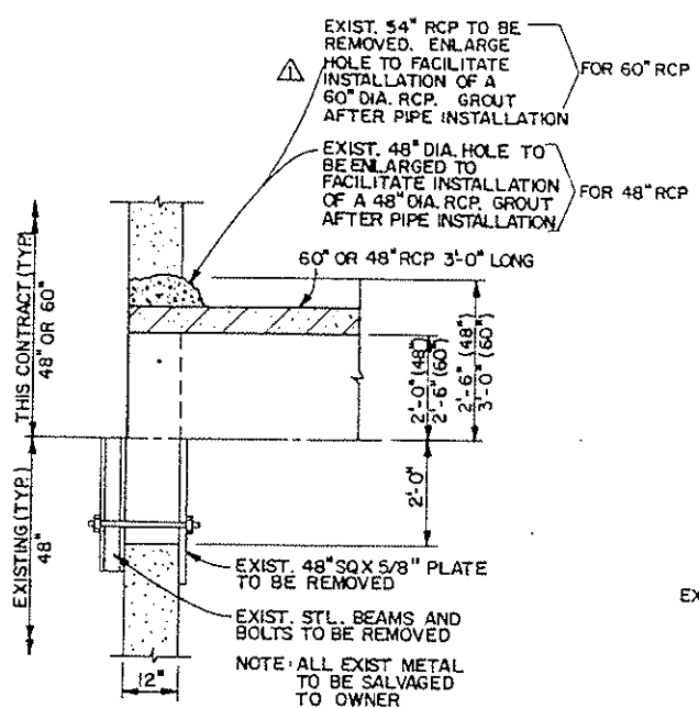
C SECTION SCALE: 1/2" = 1'-0"
